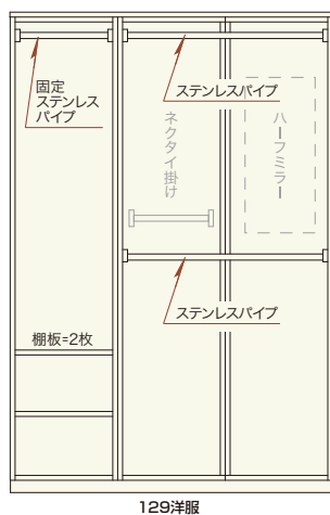
1 洋服129 W1297×D570×H1955 ¥247,700 才数54
