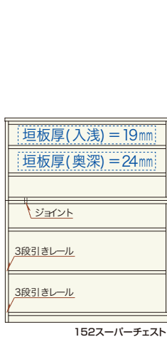
5 スーパーチェスト152(入浅) W1521×D440×H1271 ¥297,400 才数32
