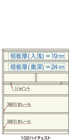
3 ハイチェスト102(入浅) W1022×D440×H1271 ¥165,400 才数22
