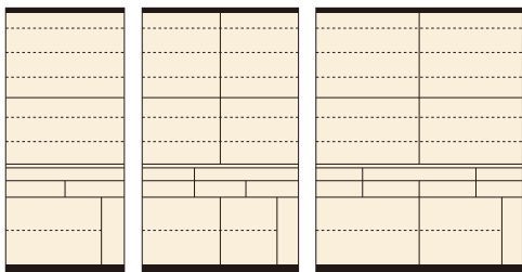
90 OPスペース 上:W818×D380×H447 下:W399×D380×H350
